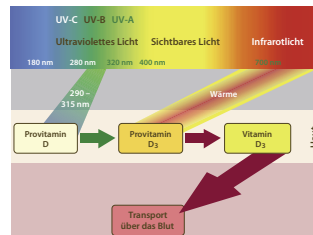
Abb.: Vitamin-D-Synthese
